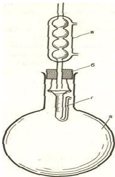
Прибор для определения содержания эфирного масла методом 1.
