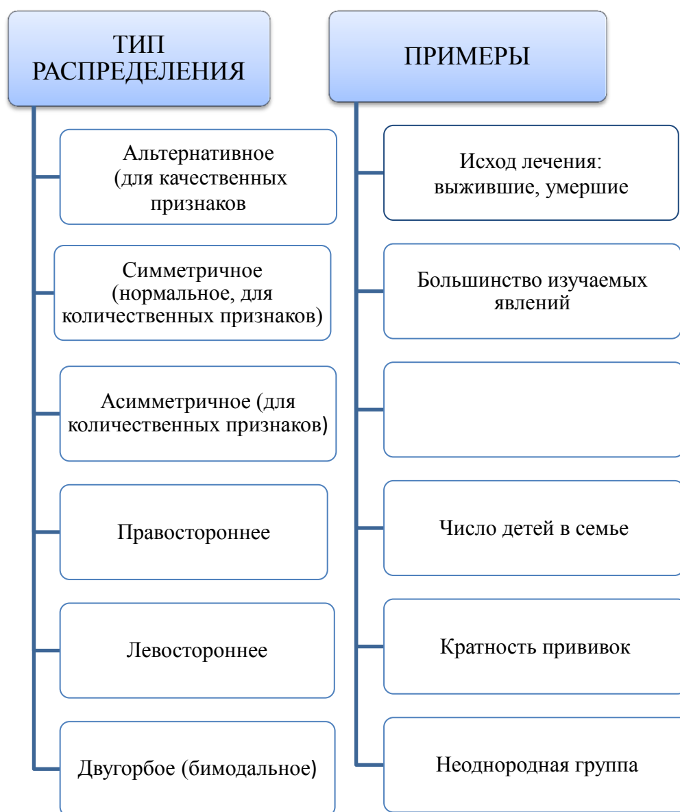
Рис. 3. Типы распределения признаков в статистической совокупности
