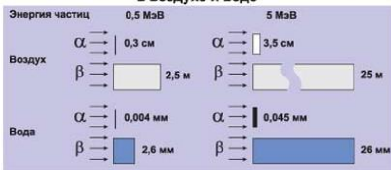
Длина пробега альфа-частиц и бета-частиц в воздухе и воде
