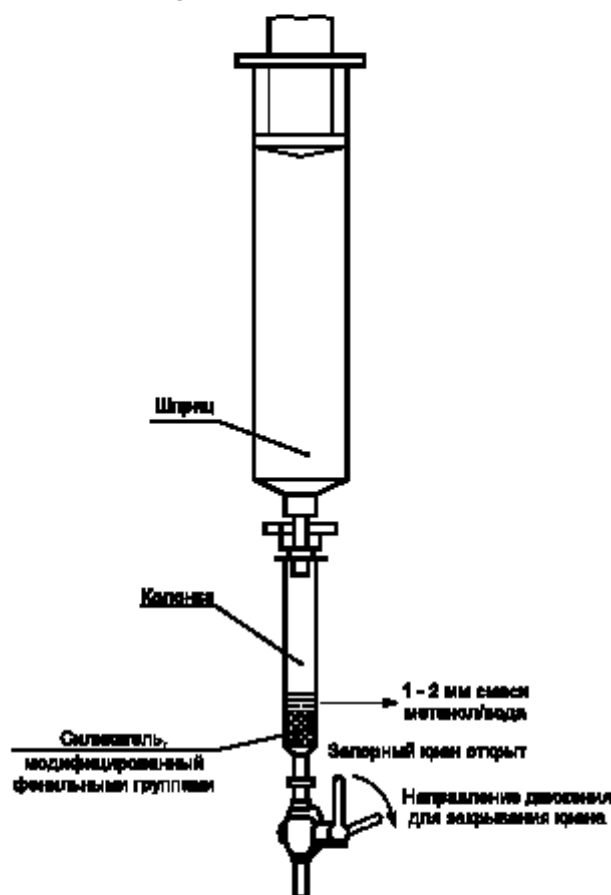
Рисунок 1 — Подготовка очистительной колонки
