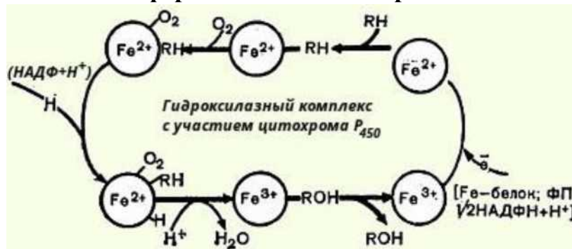
Рис. 78. Схема механизма реакции гидроксипирования в микросомах. Fe^{2*} - восстановленная форма цитохрома P-450; RH - субстрат; ФП - флавопротеид; Fe белок - белок, содержащий негеминное железо
