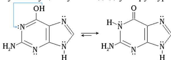
Гуанин (2-амино-6-гидроксипурин)
