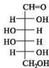
D-галактоза
