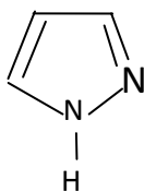
Пиразол
