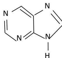
Пурин
