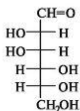
D-манноза
