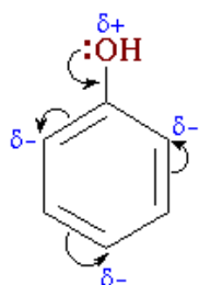
Фенол
