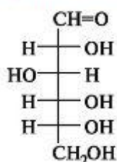
D-глюкоза
