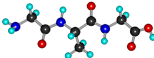
глицилаланилглицин
