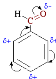
Бензальдегид
