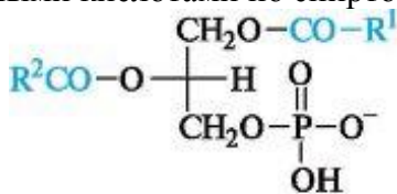
1-фосфатидовые кислоты
