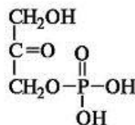
дигидроксиацетонфосфат
