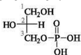
1-глицеро-3-фосфат
