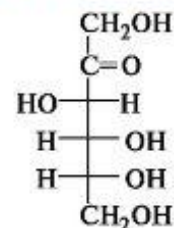
D-фруктоза
