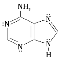
Аденин (6-аминопурин)
