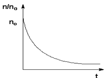
Рис. 2. Коагуляционная кривая.
