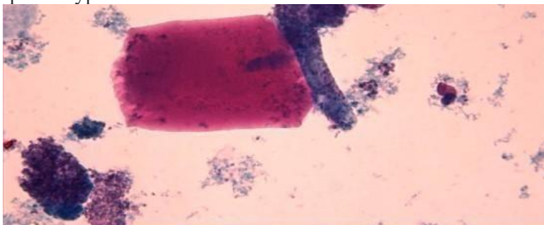
Рис.11. Псевдоцилиндр.
